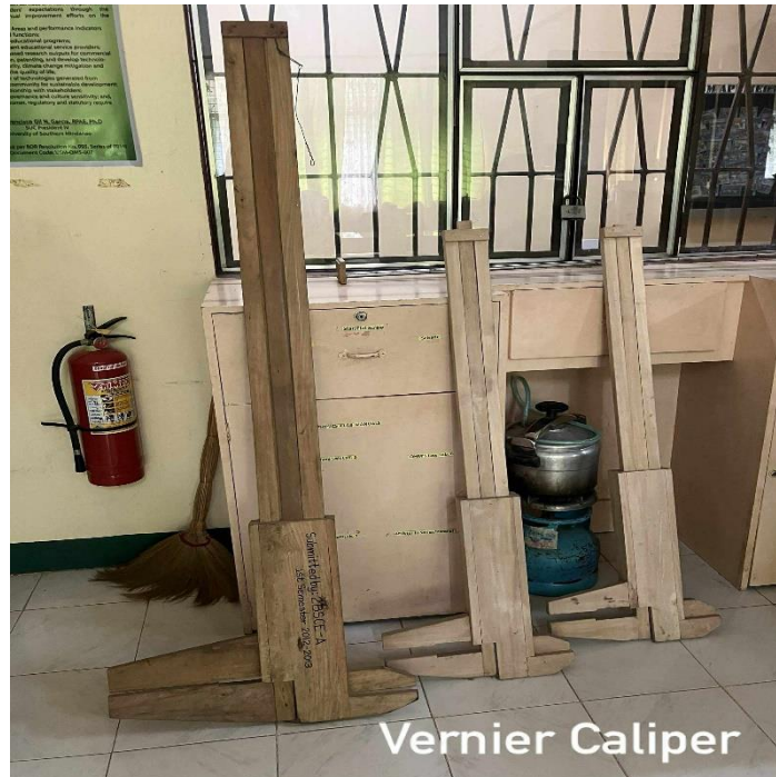
Vernier Caliper
